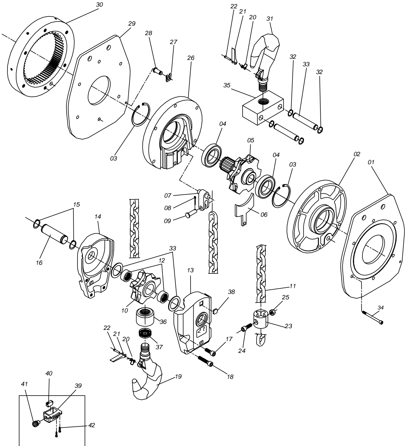
FIM DE CURSO BSEW 2T
