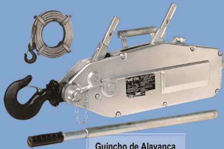
Guincho de Alavanca GA-1600 e GA-3200 kg
